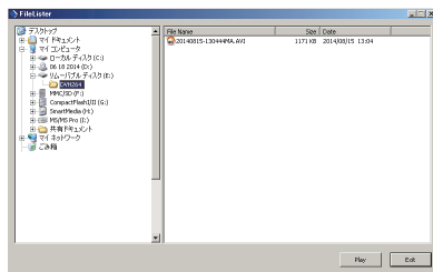
FileLister画面
